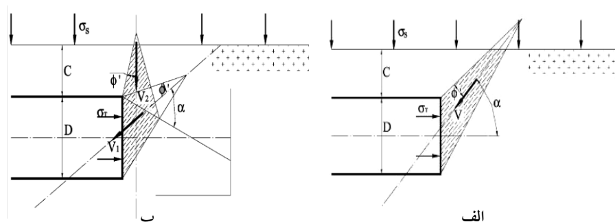
شکل ۳. مکانیزم شکست لکا-دورميو (الف) تک مخروطی (MI) (ب) دو مخروطی (MII)
