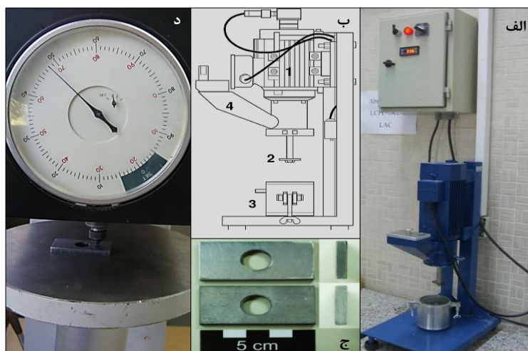
شکل ۱. الف) دستگاه سایش LCPC (دانشگاه فردوسی مشهد)، ب) شکل شماتیک دستگاه LCPC (۱) موتور، ۲) ایمپلر، ۳) ظرف نمونه، ۴) فانل تیوب (Funnel Tube)، ج) نمونه ایمپلر و د) اندازه‌گیری سختی راکول (۶۸ HRB)
