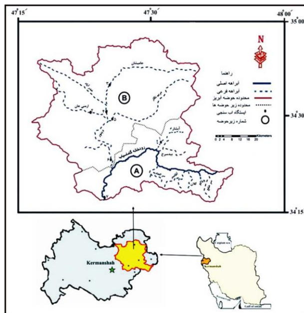
شکل ۳. موقعیت زیرحوضه‌ها و ایستگاه‌های آب‌سنجی در حوزه آبریز گاماسیاب پایین (ایستگاه‌های آب‌سنجی ۱. صحنه، ۲. خدرآباد، ۳. پیرسلمان، ۴. میانراهان، ۵. کله‌جوب، ۶. حیدرآباد، ۷. پل‌چهر) [۱۱]
