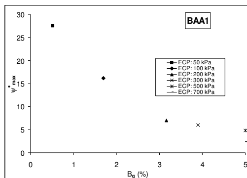
ب شکل ۱۱. رابطه زاویه اتساع مدل‌سازی در برابر نسبت شاخص شکست مارسال، الف) همه (ب) حداکثر (مثبت)
