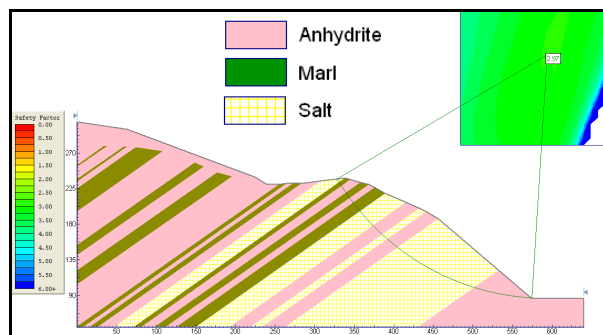
شکل ۸. شرایط پایداری دامنه در حالت بدون آبیگری (مقطع C-C)
