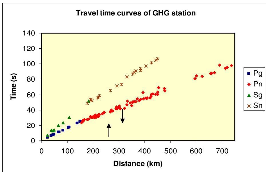
شکل ۷. نمودار زمان-مسافت موج‌های P و S در ایستگاه لرزه‌نگاری قلفزی به روش یک ایستگاهی
