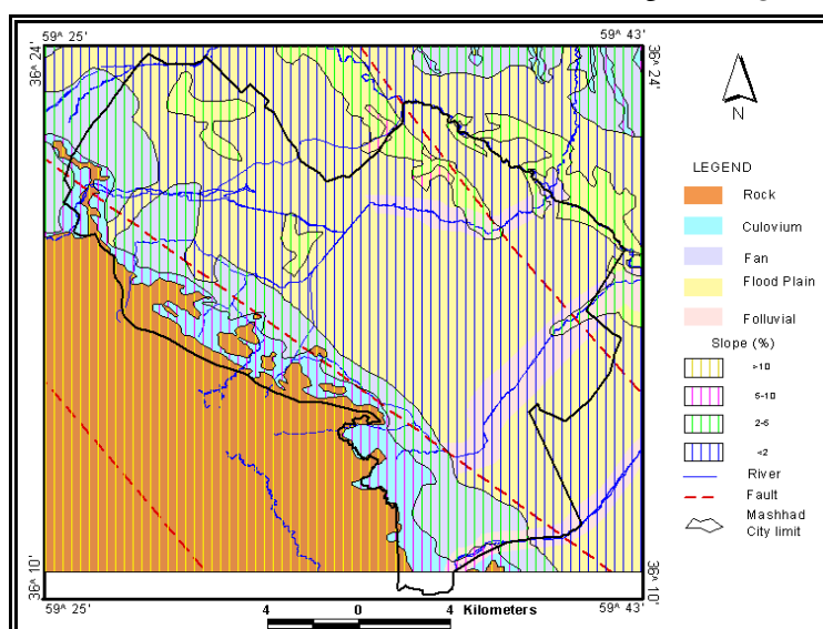
شکل ۲. نقشه پهنبندی شهر مشهد از نظر محیط رسوبی (حافظی مقدس ۱۳۸۶)
