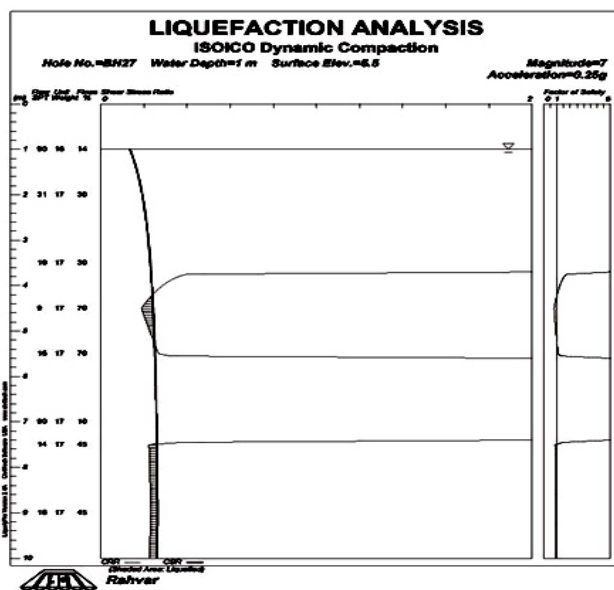
شکل ۱۱. نتیجه تحلیل روان‌گرایی گمانه Z4-BH27 با فرض وقوع زلزله به شتاب 0.25g و
