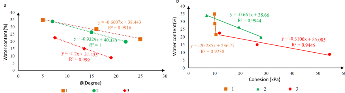
شکل ۷. تأثیر افزایش درصد رطوبت در کاهش (a) زاویه اصطکاک داخلی و (b) چسبندگی در پروفیل‌های مورد مطالعه Fig. 7. The effect of increasing moisture percentage on the reduction of a: internal friction angle and b: cohesion in the studied profiles
