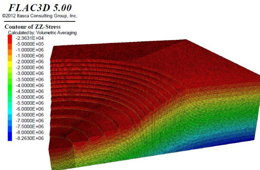
شکل ۴. توزیع تنش‌های القایی قائم در راستای Z، بعد از ایجاد پله‌های معدن
