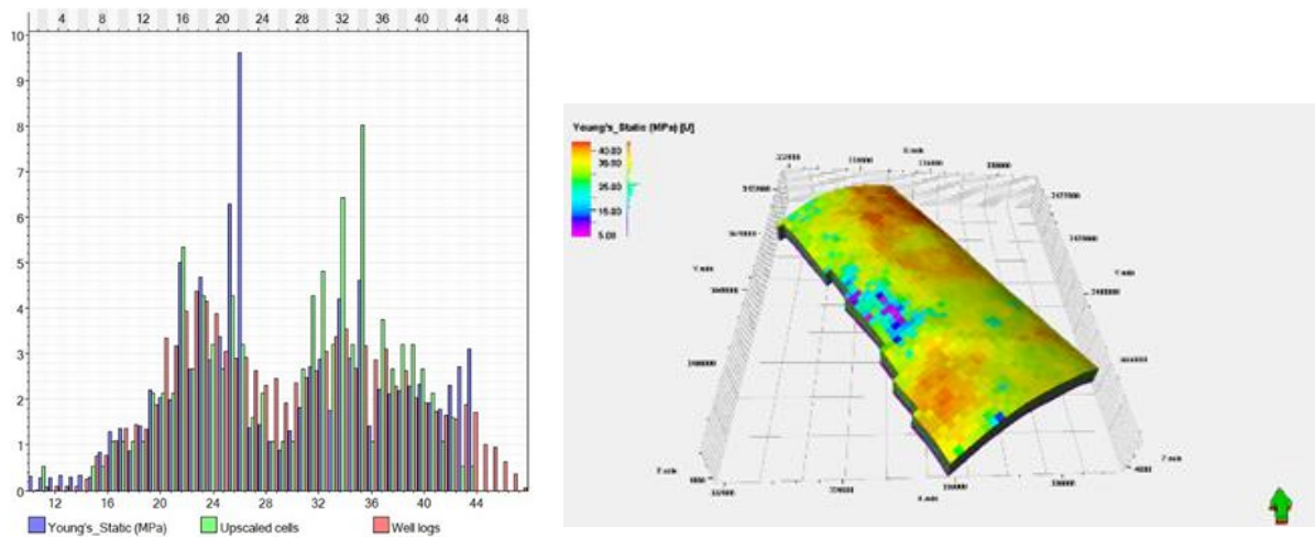
شکل ۶. مدل سه بعدی و واریوگرافی مدول یانگ استاتیکی Fig.6. Three-dimensional model and variography of static Young's modulus
