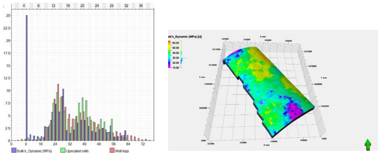
شکل ۷. مدل سه بعدی و واریوگرافی مدول بالک دینامیکی Fig.7. Three-dimensional model and variography of the dynamic bulk module
