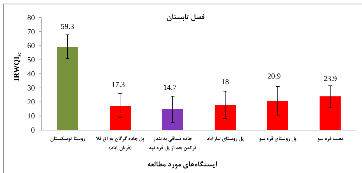
شکل ۴. مقایسه شاخص کیفی آب در ایستگاه‌های مختلف رودخانه قه‌سو در فصل تابستان ۱۴۰۰
