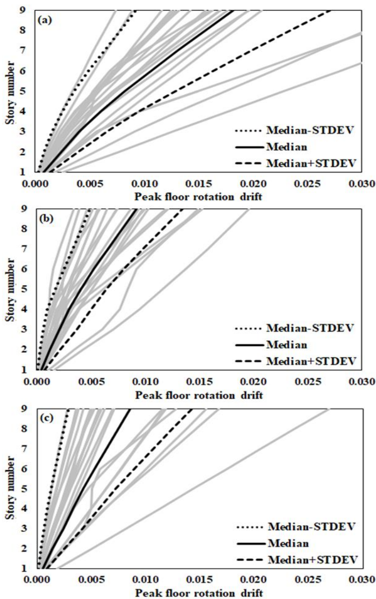
شکل ۱۳. نمودار حداکثر دررفت چرخش سقف‌های ساختمان نه طبقه در طبقات مختلف و در سطح شتاب طیفی فروریزش با e_d/A=12\% مدل آئین‌نامه‌ای، (b) مدل بالانس-۲۵٪ و (c) مدل متقارن مقاومتی
