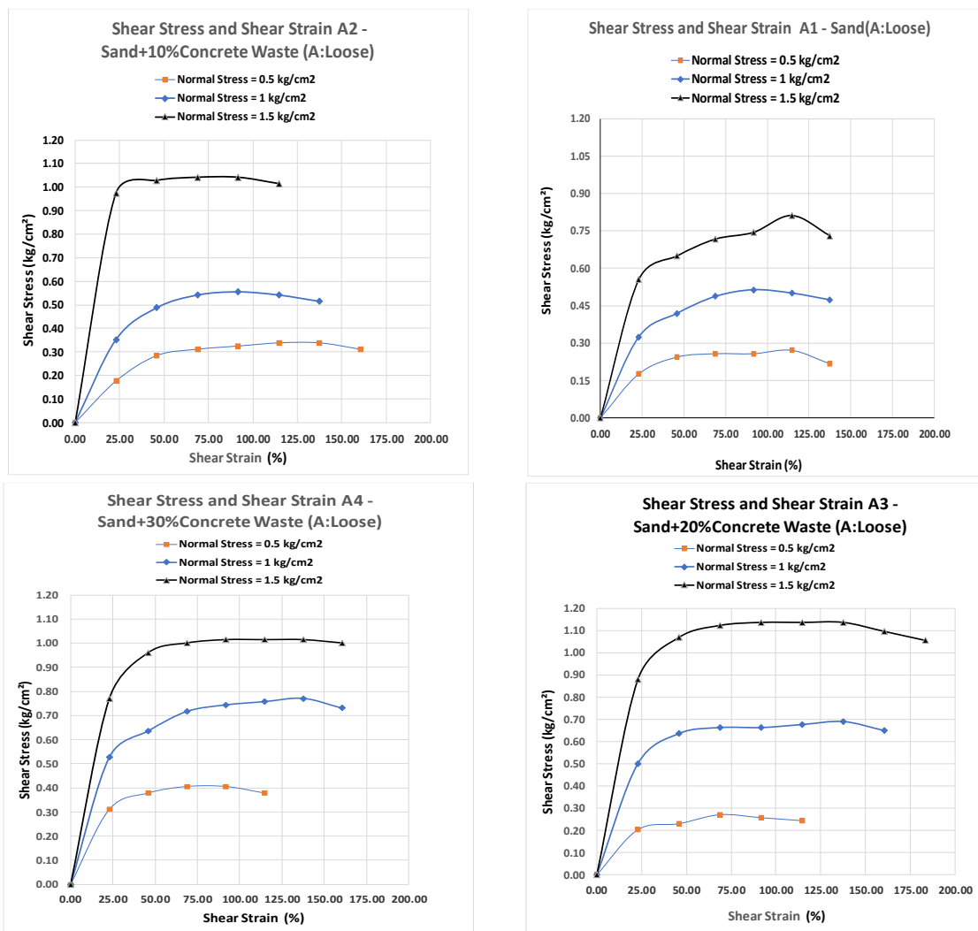
شکل ۳. نمودار تنش برشی - کرنش برشی، حالت سست (نمونه‌های سری A)
