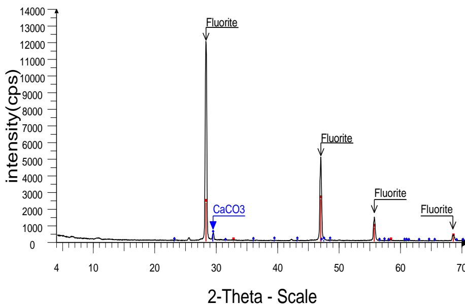
شکل ۸. نتایج حاصل از XRD نانوباریت Fig. 8. XRD results of nanobarite
