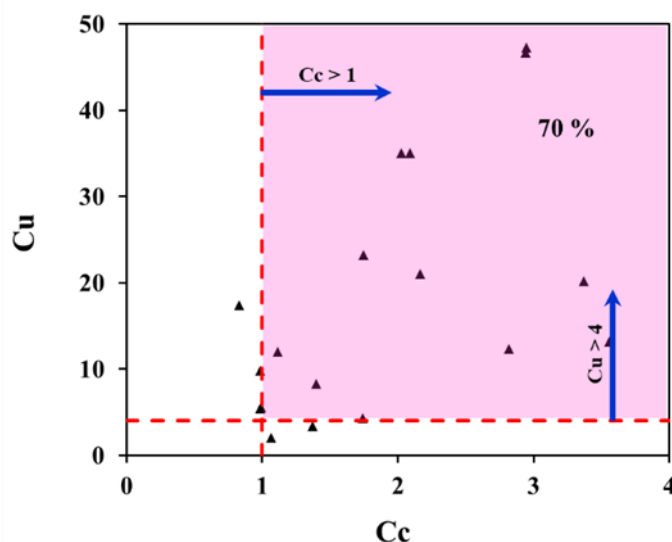
شکل ۱۴. ارزیابی ضرایب یکنواختی و انحنا پرکننده‌های سنگی استفاده شده در فعالیتهای معدنکاری
