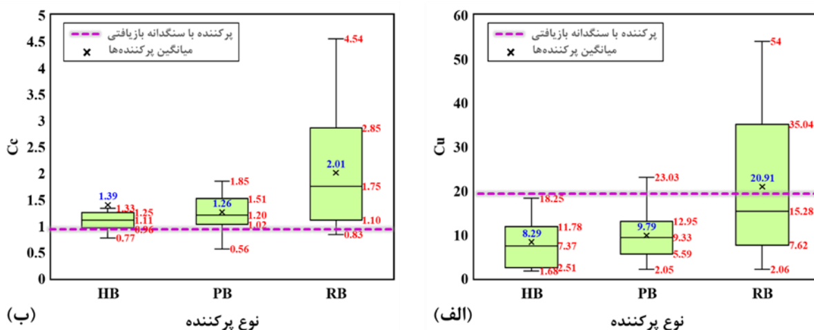
شکل ۲۰. نمودار جعبه‌ای مربوط به (الف) ضریب یکنواختی و (ب) ضریب انحنا برای پرکننده‌های هیدرولیکی، خمیری و سنگی به همراه پرکننده حاصل از سنگدانه بازیافتی
