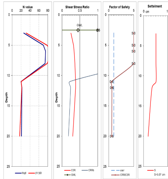
شکل ۱۸. شرایط عدد SPT، نسبت تنش برشی، وضعیت روانگرایی و نشست در گمانه شماره ۸ به روش سید و ادریس Fig. 18. The Conditions of SPT number, shear stress ratio, and liquefaction and settlement condition in borehole No.8 by Seed and Idriss method
