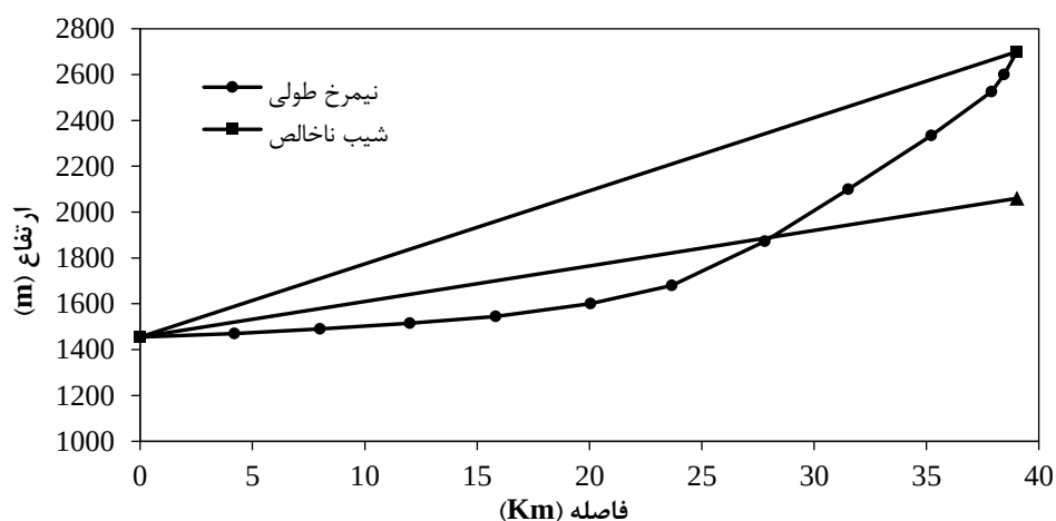
شکل ۴. نمایش نیمرخ طولی، شیب ناخالص و شیب خالص در طول مسیر رودخانه گیان Fig. 4. Longitudinal profile, real slope and apparent slope along the Gian River route
