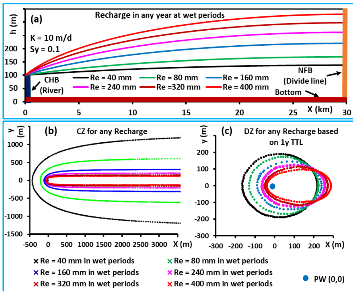
شکل 10. اثر تغذیه سطحی ( Re ): (a) سطح آب نرمال در پایان دوره‌ی تر. (b) حریم آبرگیر. (c) حریم تخلیه. خطوط زمان گذر یک ساله هستند.
