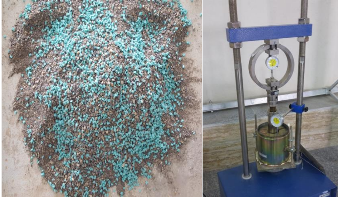
شکل ۶: مخلوط خاک و مواد EVA
