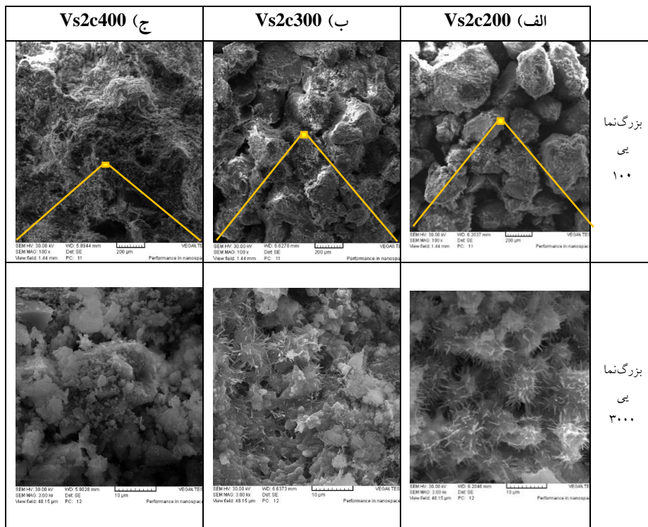
شکل ۱۳. عکس‌های SEM، تغییرات مورفولوژی ریزساختارها که در سولفات ۲٪ ایجاد شده است به ازای عیارهای مختلف سیمان تپ پنج الف) ( 200 \text{ kg/m}^3 )، ب) ( 300 \text{ kg/m}^3 )، ج) ( 400 \text{ kg/m}^3 )؛ بالا: بزرگ‌نمایی ۱۰۰ و پایین: بزرگ‌نمایی ۳۰۰۰
