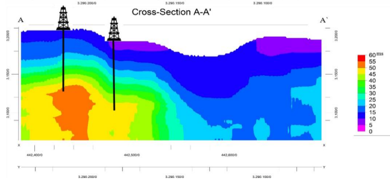
شکل ۱۳. مقطع مقاومت ویژه و پلاریزاسیون‌القایی پروفیل AA' ایجاد شده به وسیله نرم‌افزار RockWork
