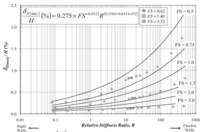
شکل ۱. تغییر شکل جانبی بر اساس سختی نسبی سیستم مهاري و ضریب اطمینان در برابر بالآمدگی (بریسون و زاپاتا) [۲۰]
