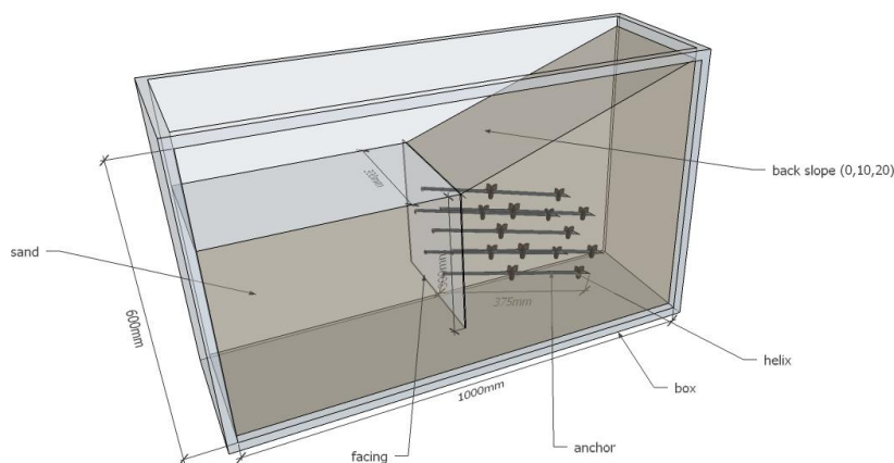
شکل ۴. چیدمان مهارها
