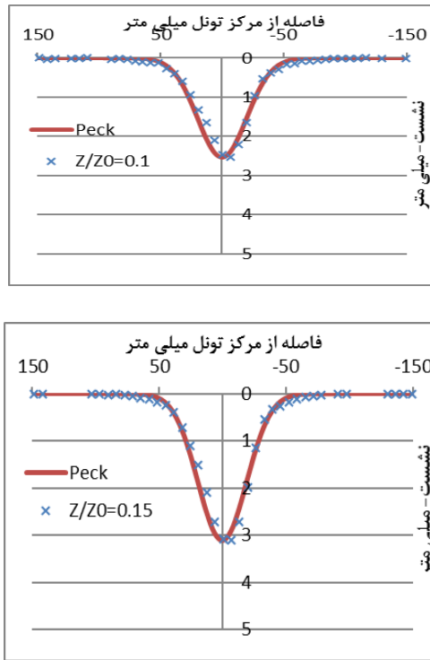
شکل ۷. نشست‌های ثبت شده و منحنی پک برازش شده برای چهار عمق مختلف برای ماسه متراکم
