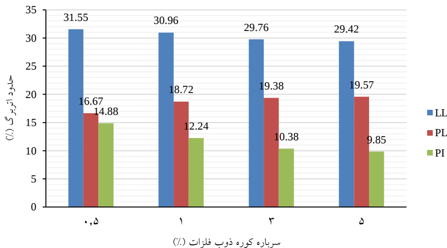
شکل ۲۴. مقایسه حدود اتبرگ و نشانه خمیری نمونه‌های با آهک ۱٪ و مقادیر مختلف سرباره
