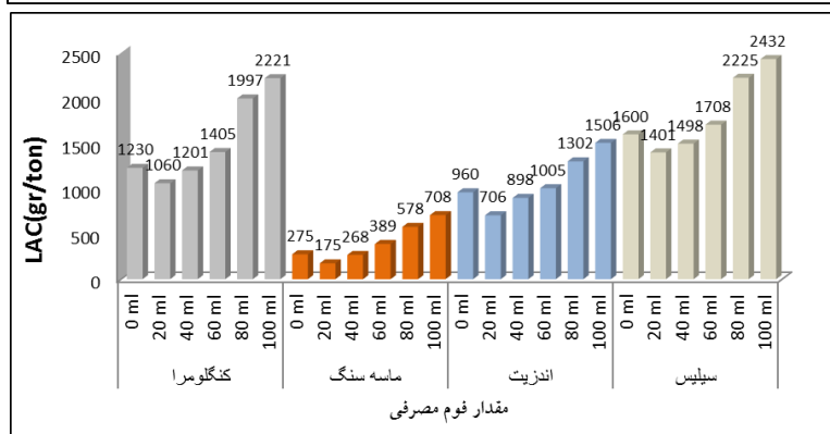
شکل ۱۳. نتایج آزمایش تعیین سایندهی مصالح فوم دار به کمک دستگاه LCPC
