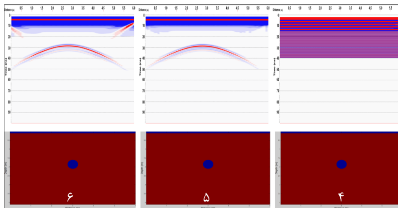
شکل ۴. بررسی تأثیر فرکانس نمونه‌برداری بر پاسخ GPR اهداف استوانه‌ای افقی توخالی در محیط میزبان از جنس خاک رس سیلتی. فرکانس نمونه‌برداری مدل ۴ برابر با ۱۰۵۹۹ مگاهرتز و در مدل‌های ۵ و ۶ رتیب برابر با ۲۳۹۷ و ۱۶۹۵۸۸ مگاهرتز است.
