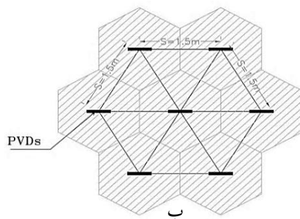
شکل ۶. الف) نمای از اجرای زهکش‌های نواری در زیر خاکریزها ب) آرایش زهکش‌ها در پلان
