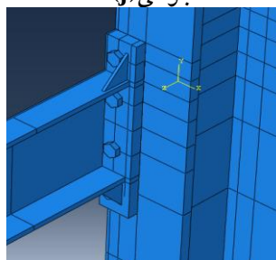
شکل ۱۰. اتصال با ورق انتهایی و لچکی (l)
