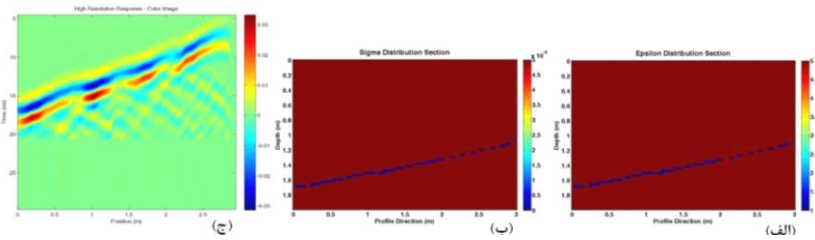
شکل ۵. الف) مقطع توزیع گذردهی دی‌الکتریک، ب) مقطع توزیع هدایت الکتریکی و ج) پاسخ GPR مدل منشور دوبعدی گرانیتی شامل یک ناپیوستگی سرتاسری
