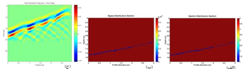
شکل ۵. الف) مقطع توزیع گذردهی دی‌الکتریک، ب) مقطع توزیع هدایت الکتریکی و ج) پاسخ GPR مدل منشور دوبعدی گرانیتی شامل یک ناپیوستگی سرتاسری
