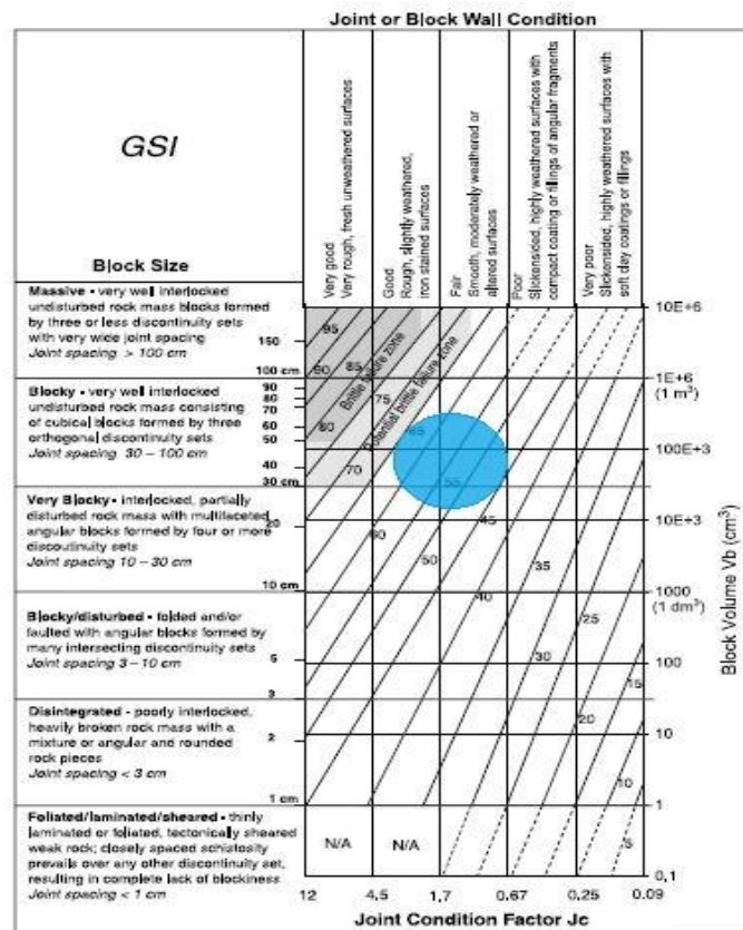
شکل ۲. نمودار کمی GSI ارائه شده به وسیله کای و همکاران (۲۰۰۴) [۹]
