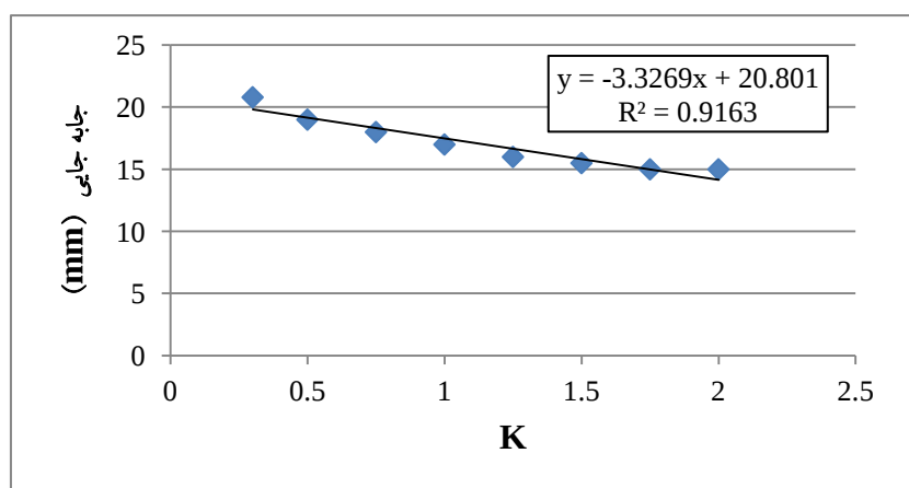
شکل ۸. نمودار تأثیر تغییرات تدریجی K بر جابه‌جایی عمودی سقف
