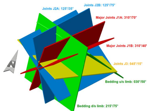
شکل ۲. نمایش سه‌بعدی ناپیوستگی‌های منطقه پروژه [۸]
