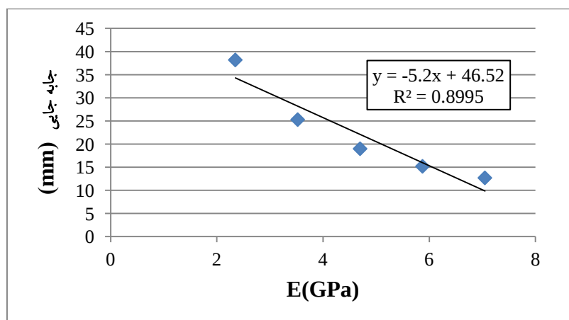
شکل ۵. نمودار تاثیر تغییرات تدریجی E بر جابه‌جایی عمودی سقف
