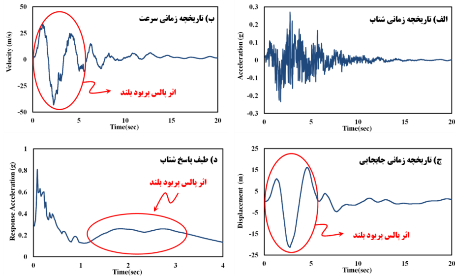
شکل ۵. الف) تاریخچه زمان شتاب، ب) تاریخچه زمان سرعت، ج) تاریخچه زمان جابه‌جایی، د) طیف پاسخ شتاب زلزله میدان نزدیک بر سنگ بستر با میرایی ۵٪
