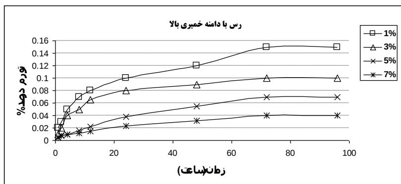
شکل ۱۲. تغییرات درصد تورم با زمان برای درصدهای مختلف افزودنی آهک به خاک رس با دامنه خمیری زیاد
