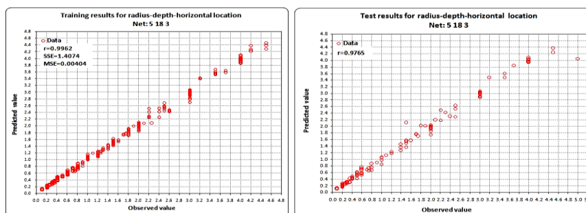
شکل ۶. نمودار پراکندگی مقادیر مشاهده‌ای پارامترهای هندسی (شعاع، عمق دفن و موقعیت افقی به‌طور هم‌زمان) در مقابل مقادیر تخمینی برای مراحل آموزش (بالا) و آزمون (پایین) با شبکه عصبی بهینه 5 \times 18 \times 3
