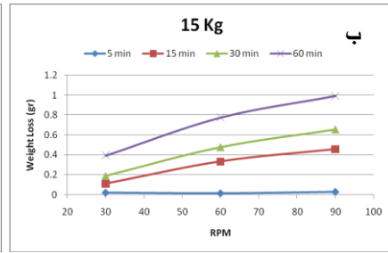
شکل ۱۲. میزان افت وزن تجمعی پیچ‌ها با تغییر در میزان سرعت چرخش برای سربارهای الف (۵، ب) ۱۵ و ج) ۲۰ کیلوگرم.
