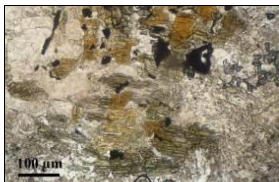
شکل ۴. عکس میکروسکوپی مقطع نازک سنگ با نور طبیعی (فتو کریست‌های آمفیبول در زمینه‌ای از شیشه)
