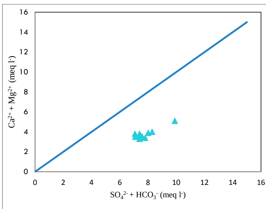
شکل ۷. نمودار Ca^{2+} + Mg^{2+} در مقابل HCO_3^- + SO_4^{2-} در نمونه های آب قنات ثلاثه
