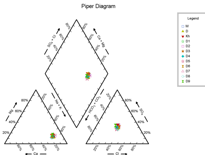
شکل ۵. نمودار پایپر نمونه‌های آب قنات Fig. 5. Piper diagram of qanat water samples
