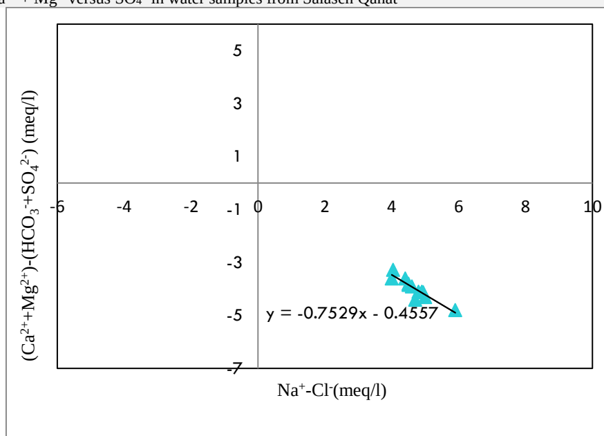
شکل ۹. نمودار \text{Na}^+ - \text{Cl}^- در مقابل (\text{Ca}^{2+} + \text{Mg}^{2+}) - (\text{HCO}_3^- + \text{SO}_4^{2-}) نمونه‌های آب قنات ثلاثه
