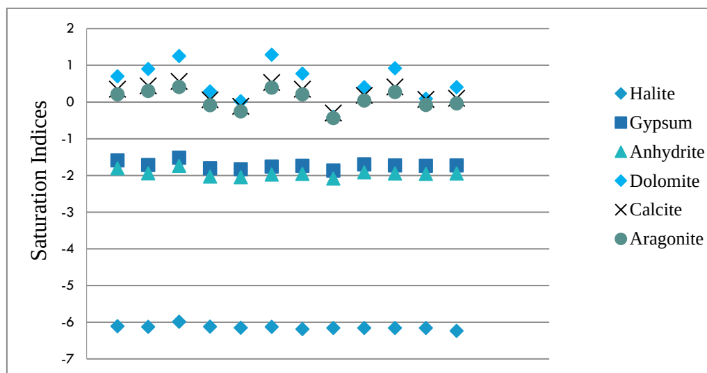
شکل ۱۱. نمودار شاخص اشباع کانی‌های مختلف در نمونه‌های آب قنات
