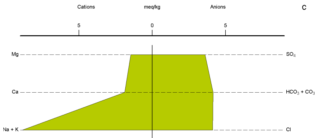
شکل ۴. نمودار استیف نمونه‌های آب قنات ثلاثه. (a) رشته خیبری، (b) رشته مند، (c) رشته دلویی. Fig. 4. Stiff diagrams of water samples from the Salaseh Qanat. a) Khaibari branch, b) Mend branch, c) Deluei branch
