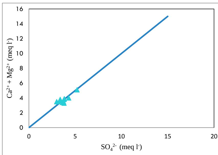
شکل ۸. نمودار \text{Ca}^{2+} + \text{Mg}^{2+} در مقابل \text{SO}_4^{2-} در نمونه‌های آب قنات ثلاثه
