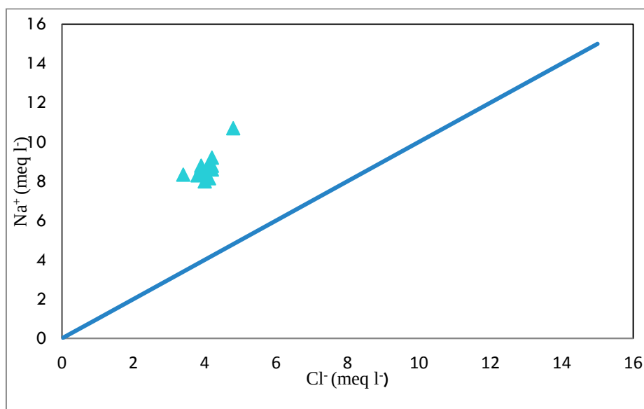
شکل ۶. نمودار کلر در مقابل سدیم نمونه‌های آب قنات ثلاثه
