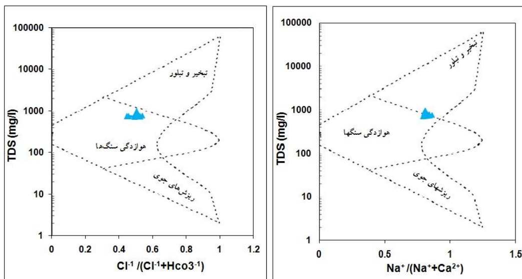
شکل ۱۰. نمودار گیبس نمونه‌های آب قنات ثلاثه گناباد
