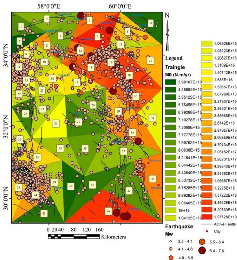
شکل ۸. تغییرات مکانی نرخ گشتاور لرزه‌ای برآوردشده به روش (IDW interpolation, power = 2) Fig. 8. Spatial variation of seismic moment rate estimated by IDW interpolation, power = 2 method
