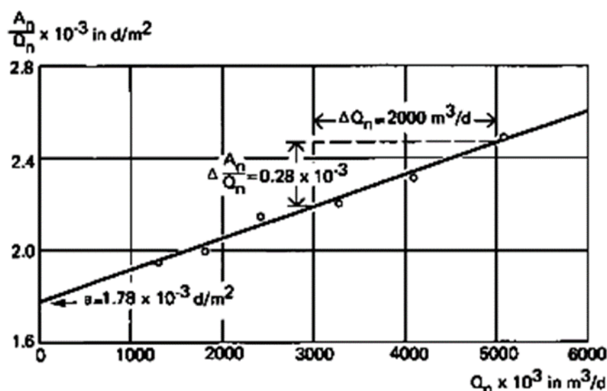
شکل ۵. روش ایدن - هیزل، داده‌های A_n/Q_n در برابر میزان Q_n (Kruseman and de Ridder, 1994)
