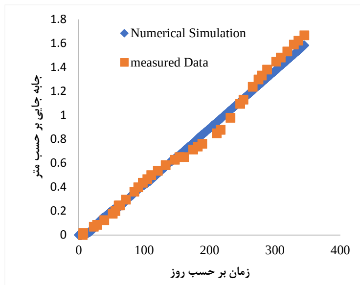
شکل ۵. مقایسه جابه‌جایی‌های محاسبه شده توسط مدل عددی و اندازه‌گیری‌های برجای برای نقطه شاهد ۰۵۱-۱۳۶۰ Fig. 5. Comparison of displacements calculated by the numerical model and in-situ measurements for reference point 051-1360
