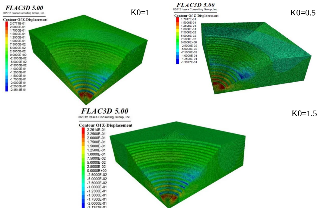
شکل ۸. کنتور جابه‌جایی‌ها در راستای Z در سناریوی سوم برای نسبت‌های تنش افقی به قائم ۱/۵ و ۰/۵ و ۱.۵ Fig. 8. Displacement contours in the Z direction in Scenario 3 for horizontal-to-vertical stress ratios of 0.5, 1, and 1.5
