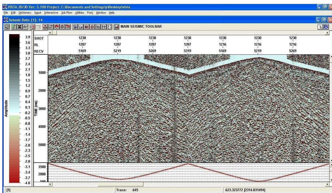
شکل ۱۶. رکورد شکل ۱۵ که تقویت AGC نیز به آن داده شده است. این شکل با استفاده از نرم افزار VISTA نمایش داده شده است
