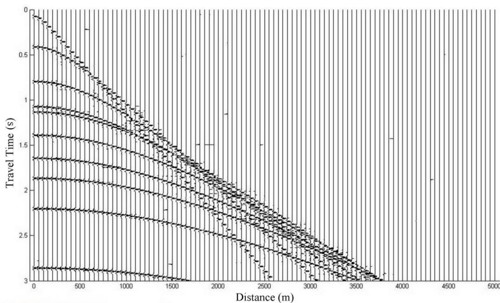
شکل ۵. رکورد چشمه مشترک مصنوعی شکل ۳ پس از اعمال فیلتر میانی دو بعدی با طول ۹ نقطه که با استفاده از نرم‌افزار MATLAB ساخته شده است. همان‌طور که در این شکل ملاحظه می‌شود هنوز مقدار کمی نوفه‌ی تصادفی در این رکورد وجود دارد
