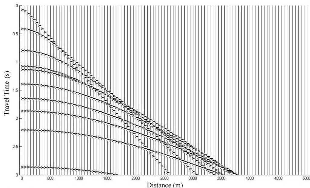
شکل ۲. رکورد لرزه‌ای چشمه مشترک مصنوعی ساخته شده با استفاده از مدل سرعت و ضخامت جدول ۱. در این رکورد مصنوعی که با استفاده از نرم‌افزار MATLAB ساخته شده است و در آن ۱۰۰ رد لرزه به فاصله‌ی ۵۰ متر از یکدیگر قرار دارند، زمان نمونه‌برداری ۲ میلی ثانیه می‌باشد
