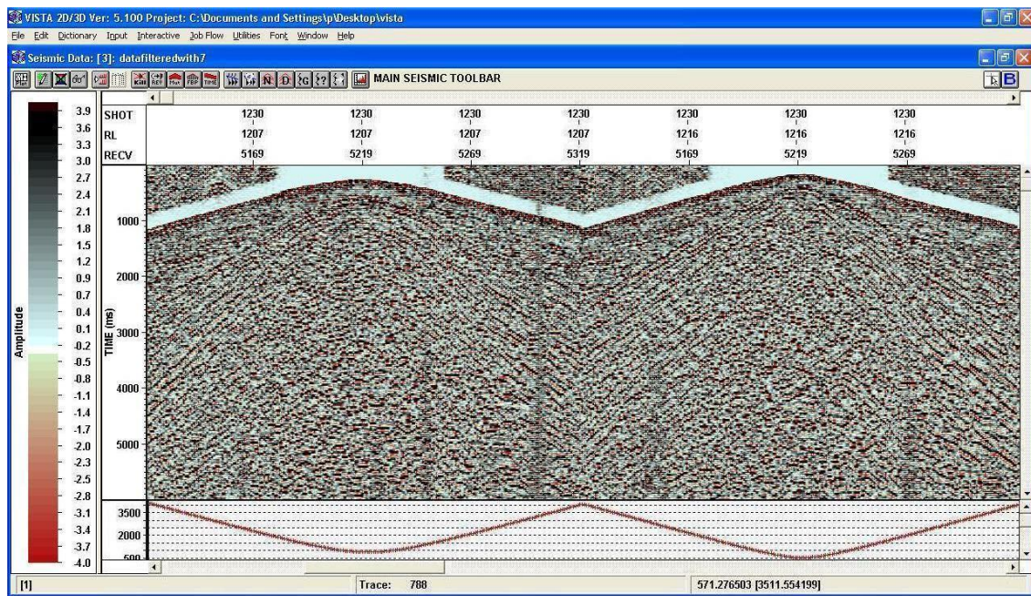
شکل ۱۷. رکورد شکل ۱۶ پس از اعمال فیلتر میانی دو بعدی با طول ۷ نقطه و تقویت AGC. این شکل با استفاده از نرم‌افزار VISTA نمایش داده شده است
