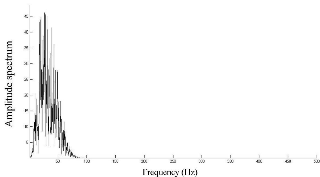
شکل ۷. طیف دامنه‌ی مربوط به رد لرزه‌ی سی‌ام شکل ۲ که هنوز نوفه‌ی تصادفی به داده‌ی مصنوعی اضافه نشده است و با استفاده از نرم‌افزار MATLAB ساخته شده است
