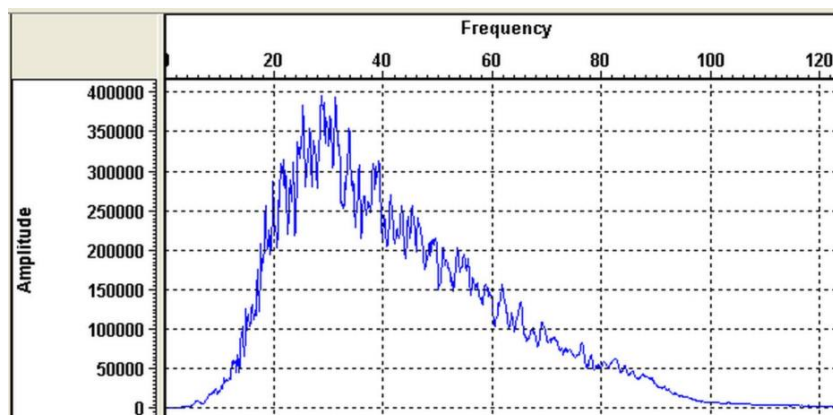
شکل ۲۴. طیف دامنه‌ی متوسط مقطع برانبارش شده‌ی واقعی پیش از اعمال فیلتر میانی دو بعدی. این شکل با استفاده از نرم‌افزار VISTA نمایش داده شده است
