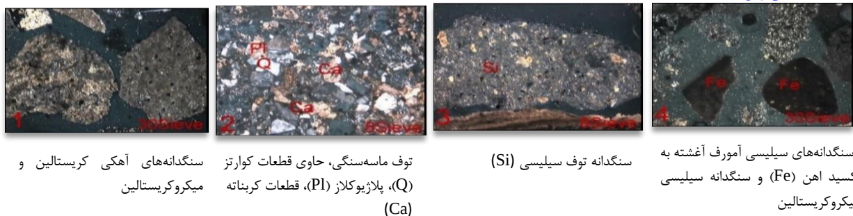
شکل ۳. مقطع میکروسکوپی سنگدانه ها براساس ASTM C295 Fig. 3. Microscopic section of aggregates according to ASTM C295
