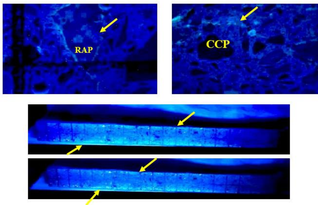
شکل ۱۰. واکنش ASR بر روی سطح صیقلی شده نمونه زیر نور UV با استفاده از آزمایش محلول اورانیل استات
