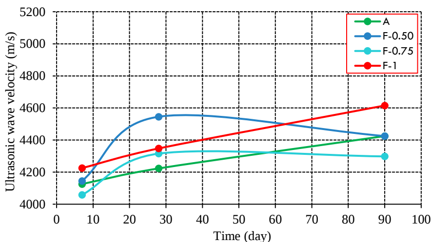
شکل ۱۴. سرعت سیر امواج اولتراسونیک در نمونه‌های حاوی نانوفلوریت
