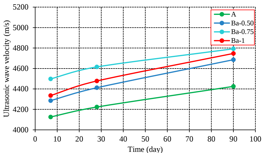
شکل ۱۳. سرعت سیر امواج اولتراسونیک در نمونه‌های حاوی نانوباریت
