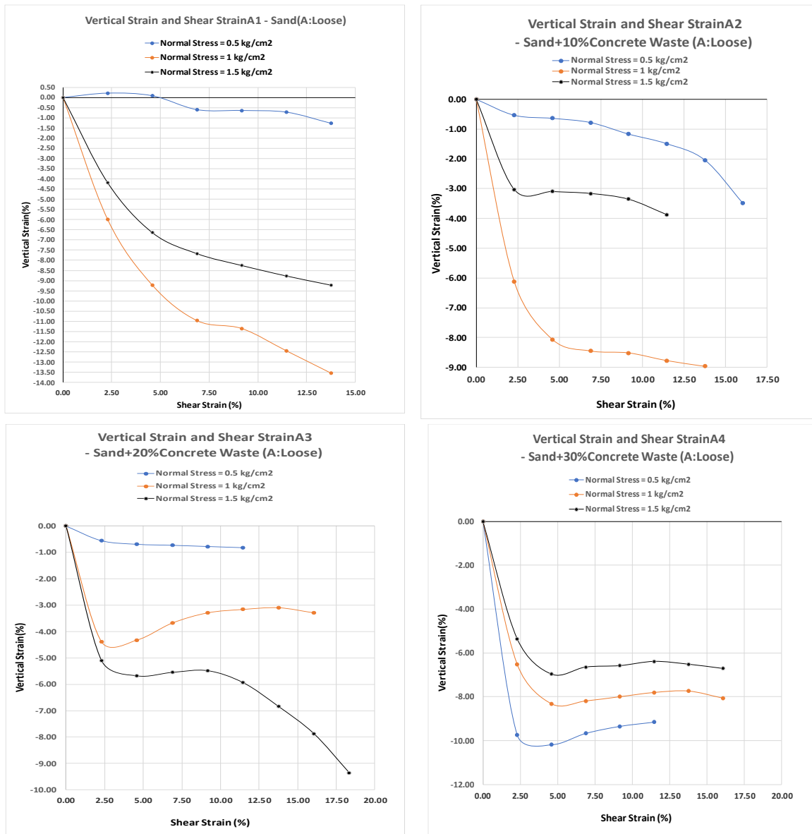
شکل ۴. نمودار کرنش برشی - کرنش قائم، حالت سست (نمونه‌های سری A) Fig. 4. Vertical Strain - Shear Strain diagram for loose sand (samples A)
