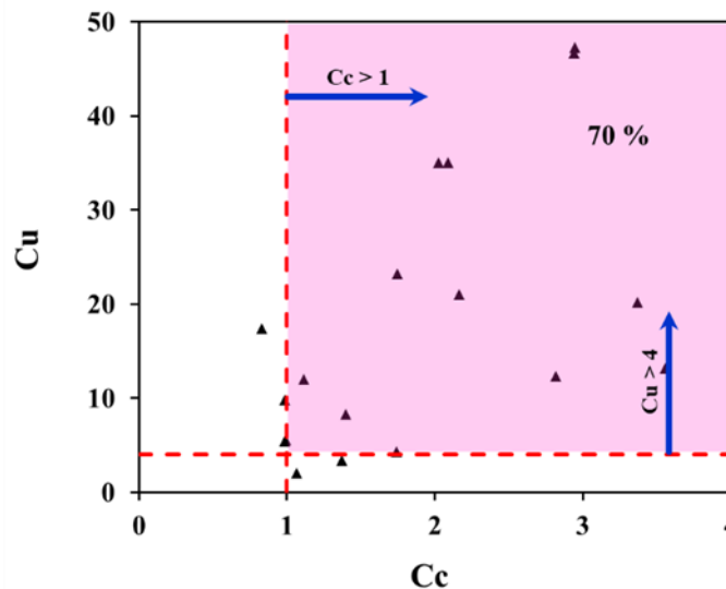
شکل ۱۴. ارزیابی ضرایب یکنواختی و انحنا برای پرکننده‌های سنگی استفاده شده در فعالیتهای معدنکاری
