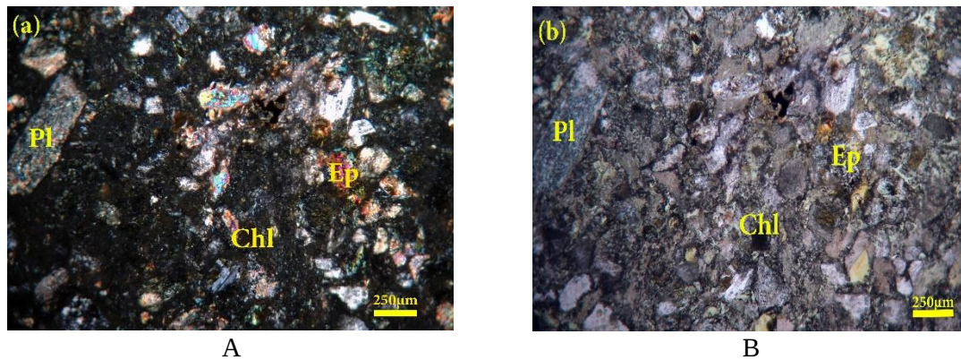
شکل ۱. پتروگرافی سنگدانه مصالح پایه (A: نور طبیعی و B: نور پلاریزه) Fig. 1. Aggregate petrography of the base material (A: normal light, B: Polarized light)
