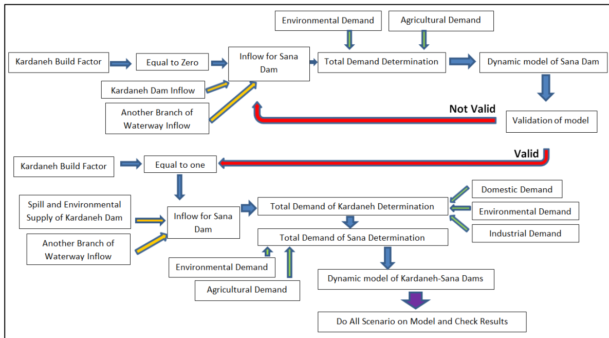
شکل ۲. فلوچارت کلی مدل‌سازی سدهای کارنده-سنا
